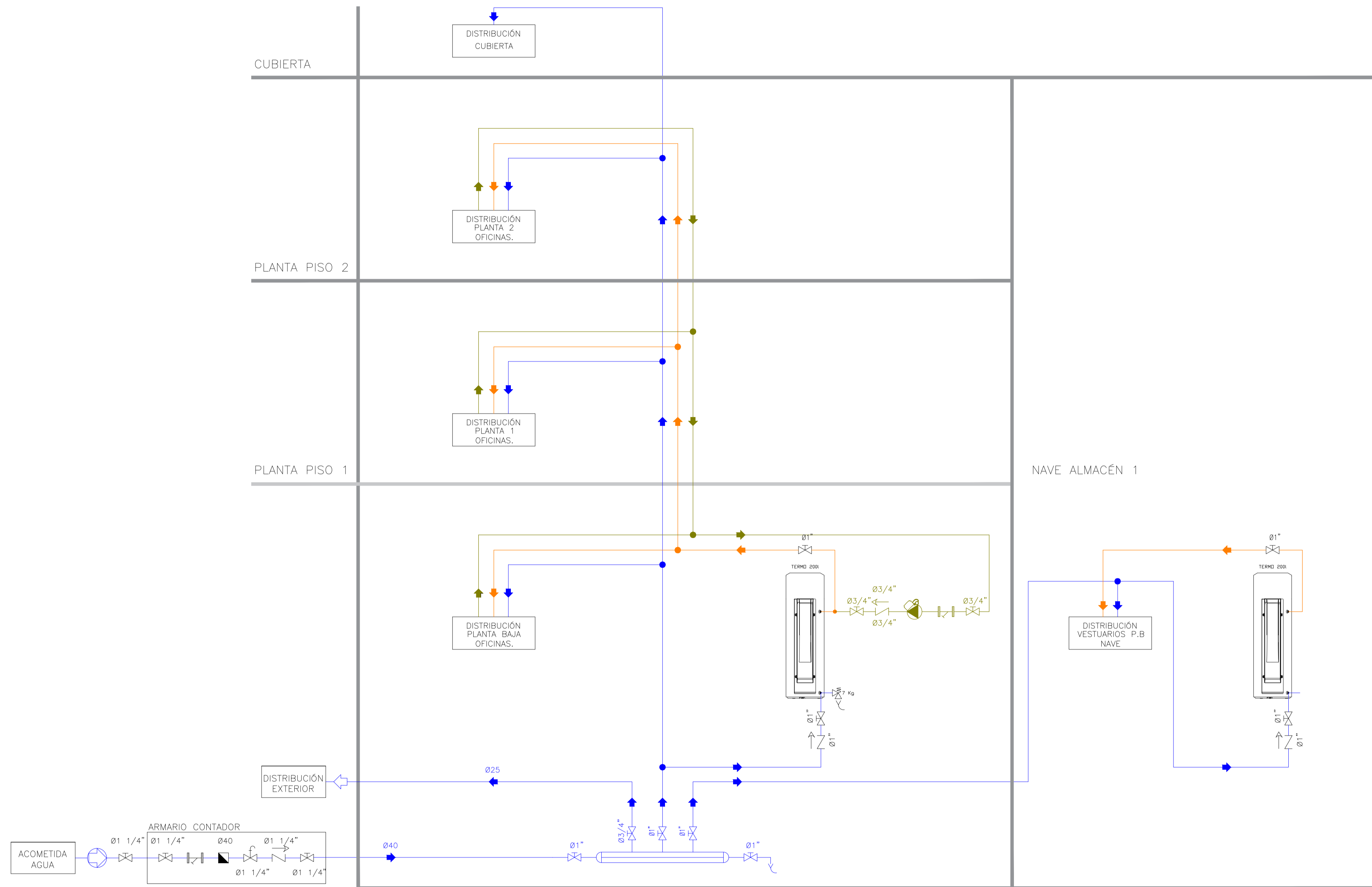
DIAGRAMA DE PRINCIPIO FONTANERIA
